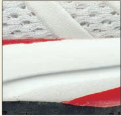
C.M. E.V.A. Compression Moulded E.V.A. E.V.A. – dieses Verfahren sorgt für eine leichte, gepolsterte Zwischensohle, die widerstandsfähiger gegen Abnutzung ist.
